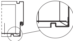
Nagel-/ Dübelanker- Befestigung
