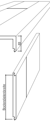
TSK 1x eingeschlagen ohne Träger inkl. Setzstufe
